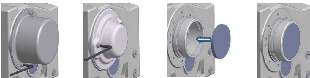
Fig. 14: Montering av deksler alternativ SH, alternativ H og alternativ H66
