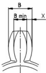
Figur 29: Måling av tanntykkelsen på klokoblingen ROTEX®
