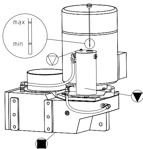
Fig. 37: Tapp-/parallelgir med oljenivåbeholder
