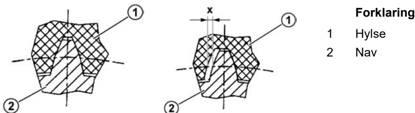
Figur 30: Måling av tannhylseslitasjen på den buede tannkoblingen BoWex®
