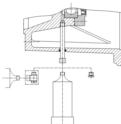
Fig. 22: Montering av fettopsamlingsbeholderen
