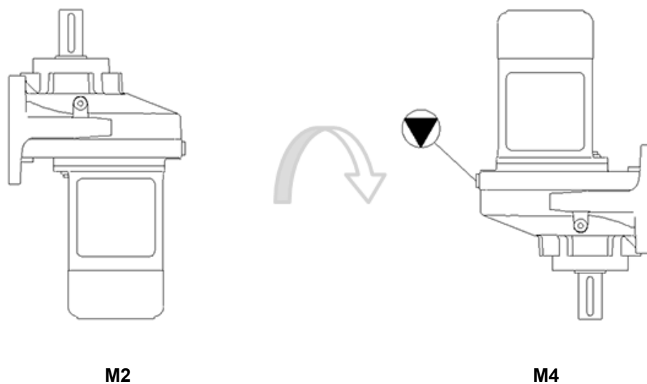
Fig. 35: Oljenivåmåling SK 071.1 – SK 371.1
