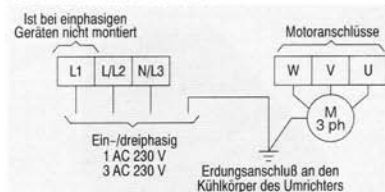
Bild 3: Netz- und Motoranschlüsse
