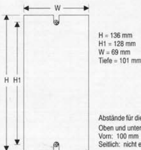
Bild 1: Schema für die Montage
